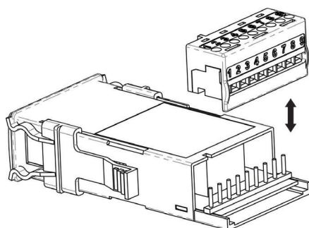
Fig. 02 - Extracción del conector trasero
