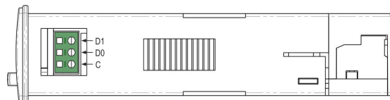
Fig. 03 – Conexiones de la comunicación serial RS485
